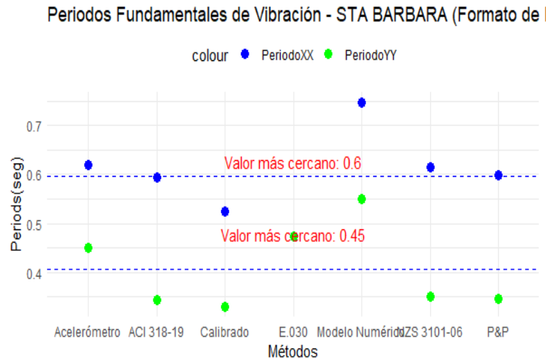
Figura 9. Valores de T(s) para diferentes metodologías de análisis sísmico en edificio STA BARBARA
