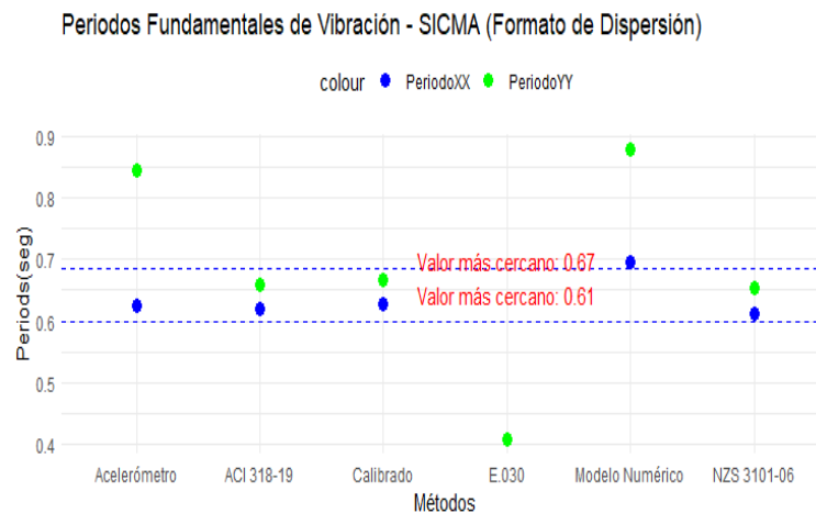
Figura 6. Valores de T(s) para diferentes metodologías de análisis sísmico en edificio SICMA.
