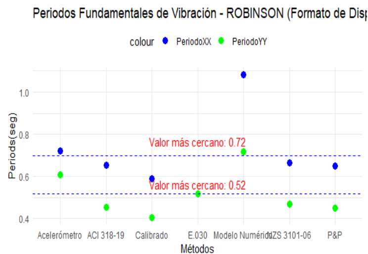
Figura 8. Valores de T(s) para diferentes metodologías de análisis sísmico en edificio ROBINSON
