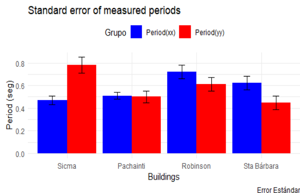
Figura 5. Error estándar de Periodos Naturales de Vibración obtenidos.
