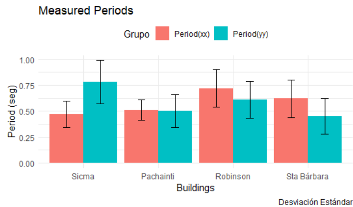
Figura 4. Periodos Naturales de Vibración obtenidos.
