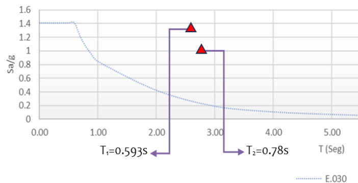
Figura 6. Influencia de la variación de periodo en espectro de aceleraciones.
