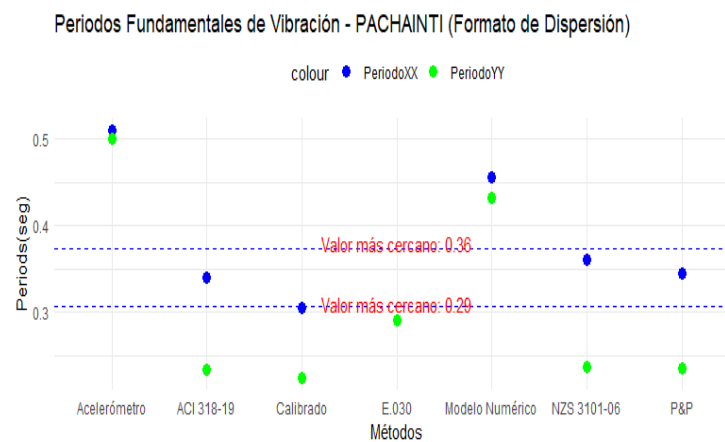
Figura 7. Valores de T(s) para diferentes metodologías de análisis sísmico en edificio PACHAINTI
