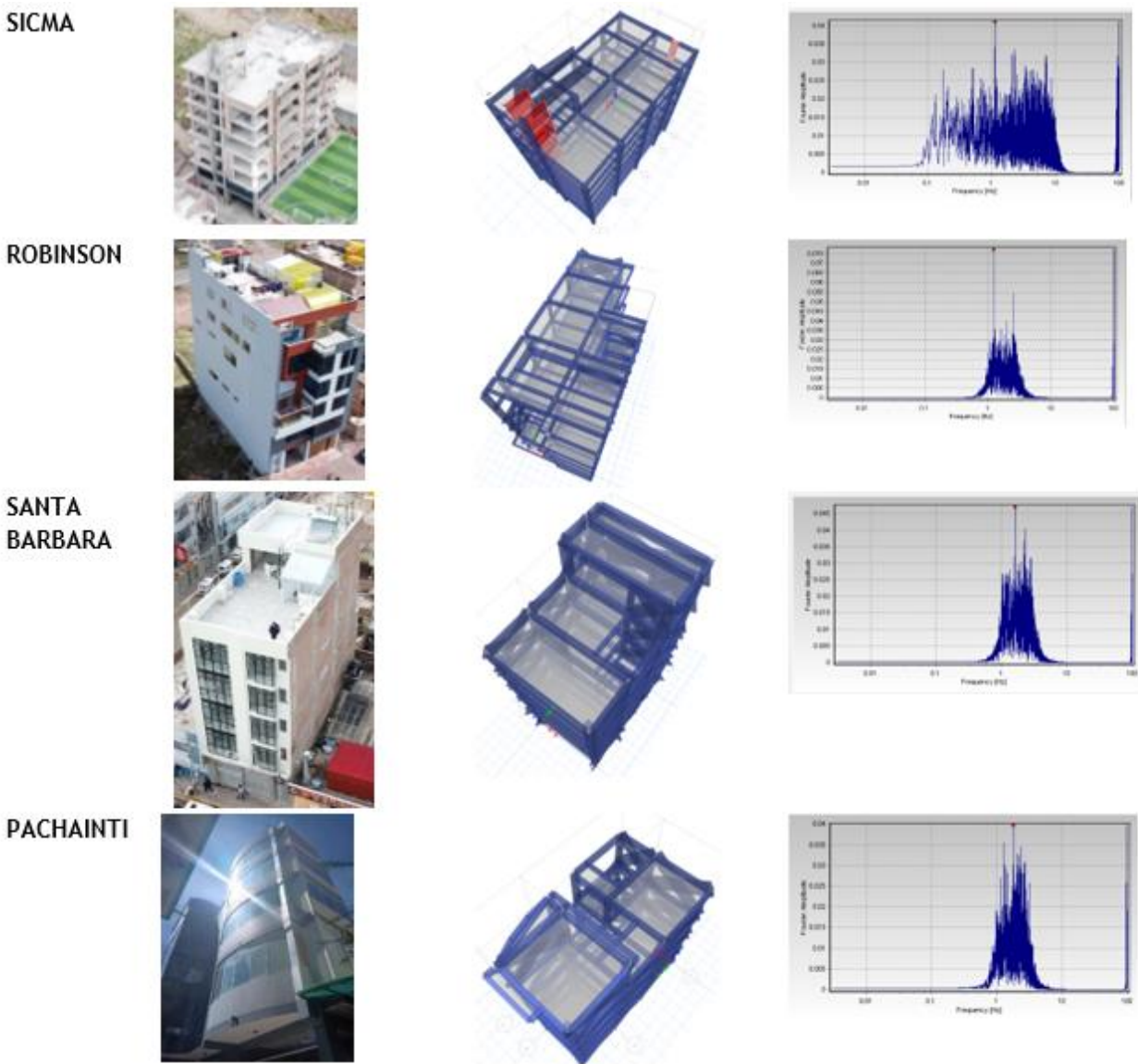
Figura 1. Edificaciones estudiadas y su representación numérica, de izquierda a derecha: nombre del edificio, foto real del edificio, modelo numérico en Etabs, resultado del periodo predominante de la edificación medido con los sensores.
